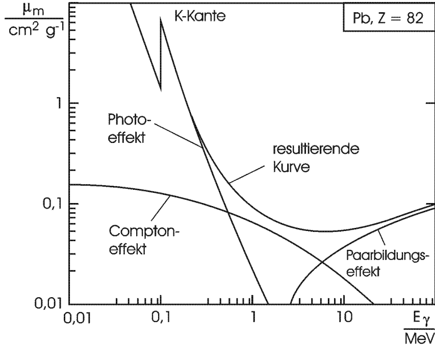
Abbildung 7: Massenschwächungskoeffizient \mu_m von Blei ( Z = 82 ) als Funktion der Quantenenergie E_\gamma .
