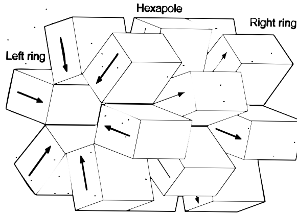
Abbildung 9: Kompakt-ECR mit vollpermanenten Magnetfeldkomponenten. Die Pfeile geben die Magnetisierungsrichtungen der einzelnen Magnetblöcke an.
