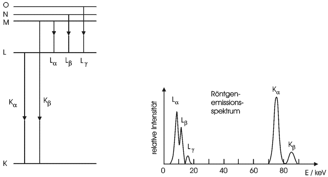
Abbildung 4: Entstehung charakteristischer Röntgenstrahlung bei der Auffüllung von Innerschalenlücken und prinzipielles Erscheinungsbild von Röntgenspektren.
