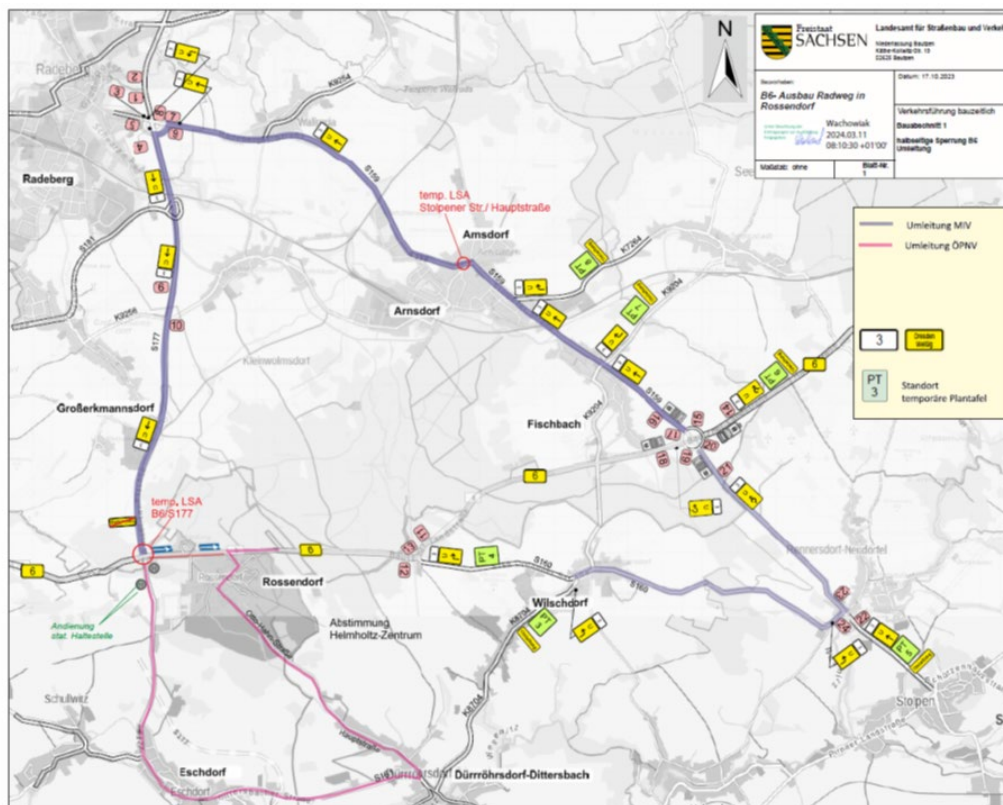
Umleitungsplan Teilabschnitt 5 – halbsseitige Sperrung B 6
